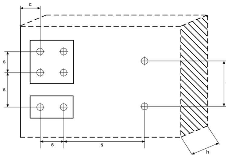
Anordnung Randabstände und Achsabstände in Beton
